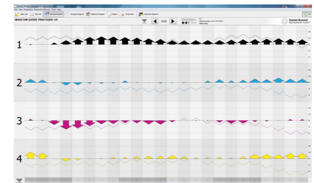
Recomendaciones de regulación con equilibrio de grises/color para cada zona de entintado y unidad de impresión
